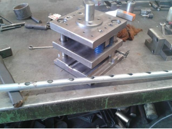
Manuel-Otomatik Sürücülü BORU Delme Kalıbı
