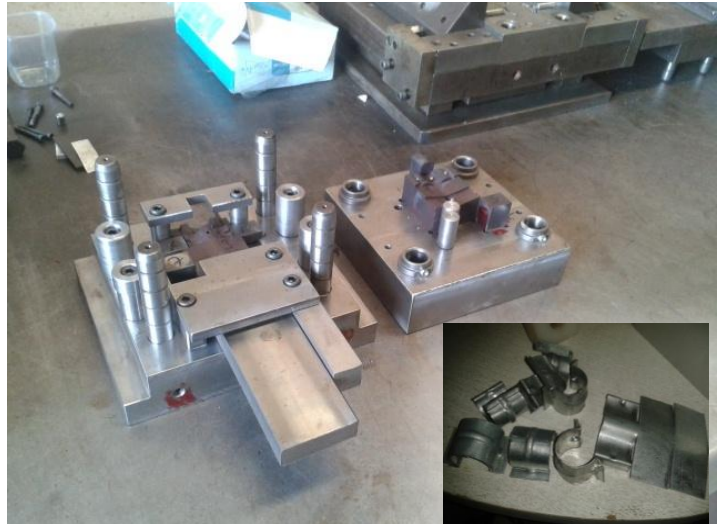
Adımlı Kombine kesimli+bükümlü SAÇ KELEPÇE Kalıbı
